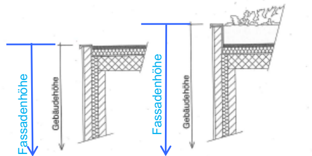
Darstellung Messweise Gebäudehöhe resp. Fassadenhöhe bei Flachdächern (Zürcher Planungs- und Baurecht, Band 2 S. 919, Fritsche, Bösch, Wipf)
