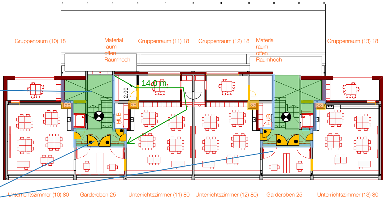
Obergeschoss
